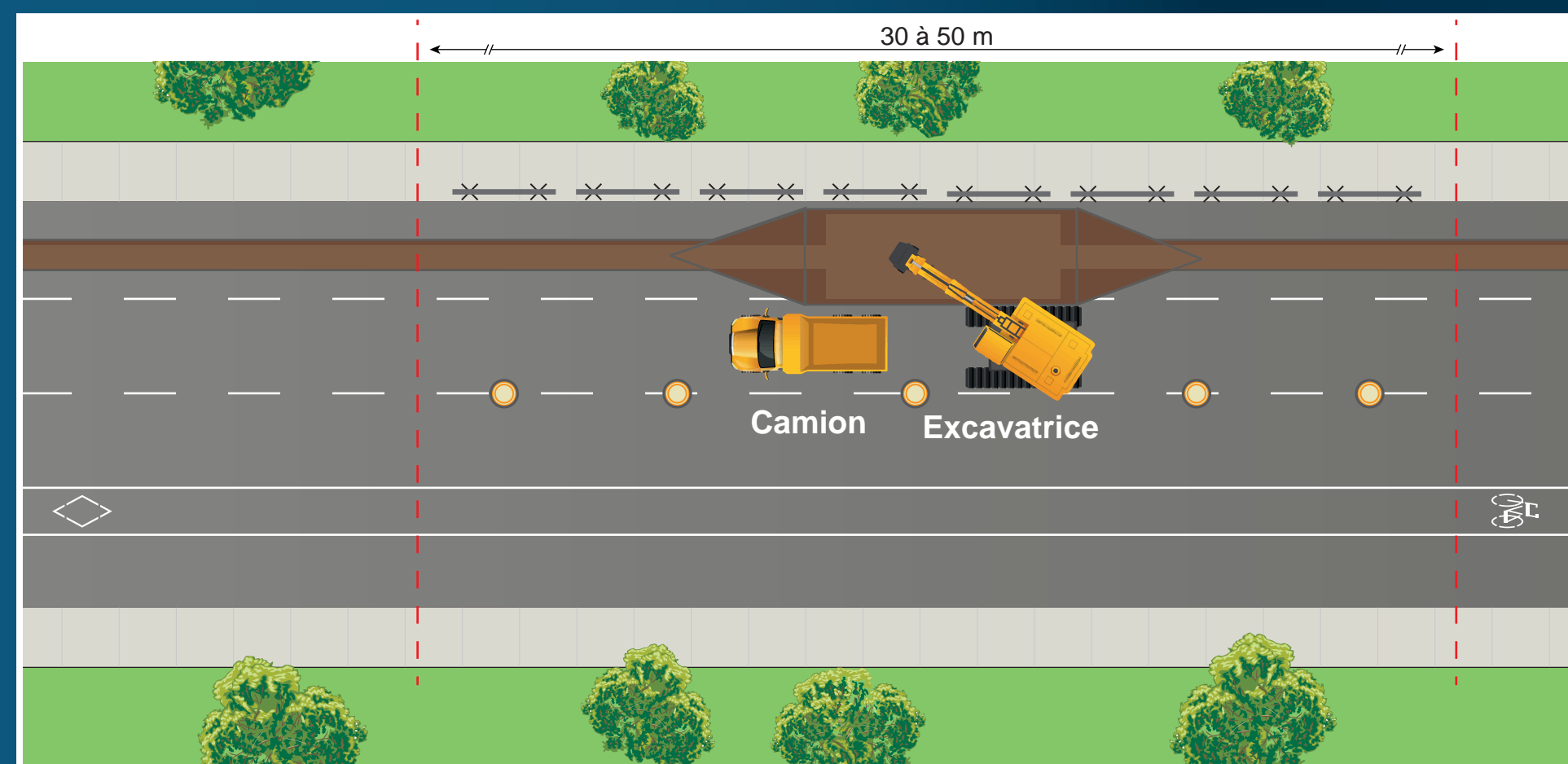
Étape 1 – Excavation et étançonnement
