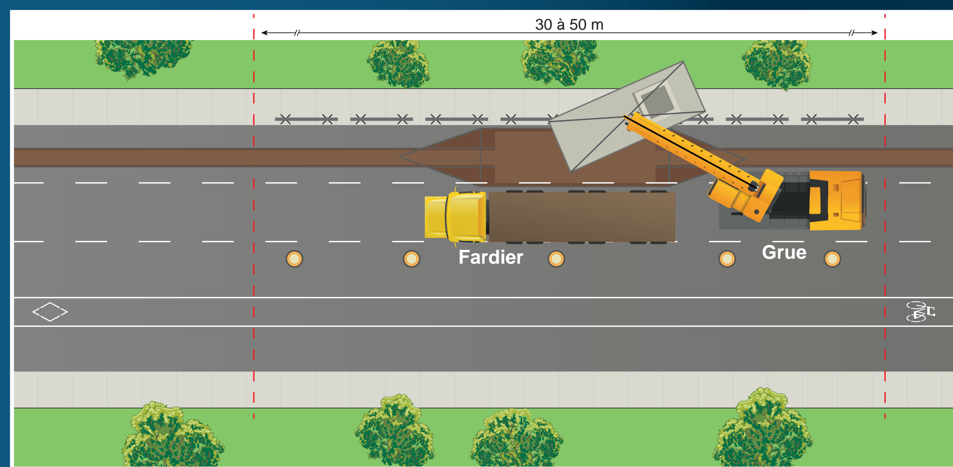
Étape 2 – Livraison et installation d'une chambre de jonction
