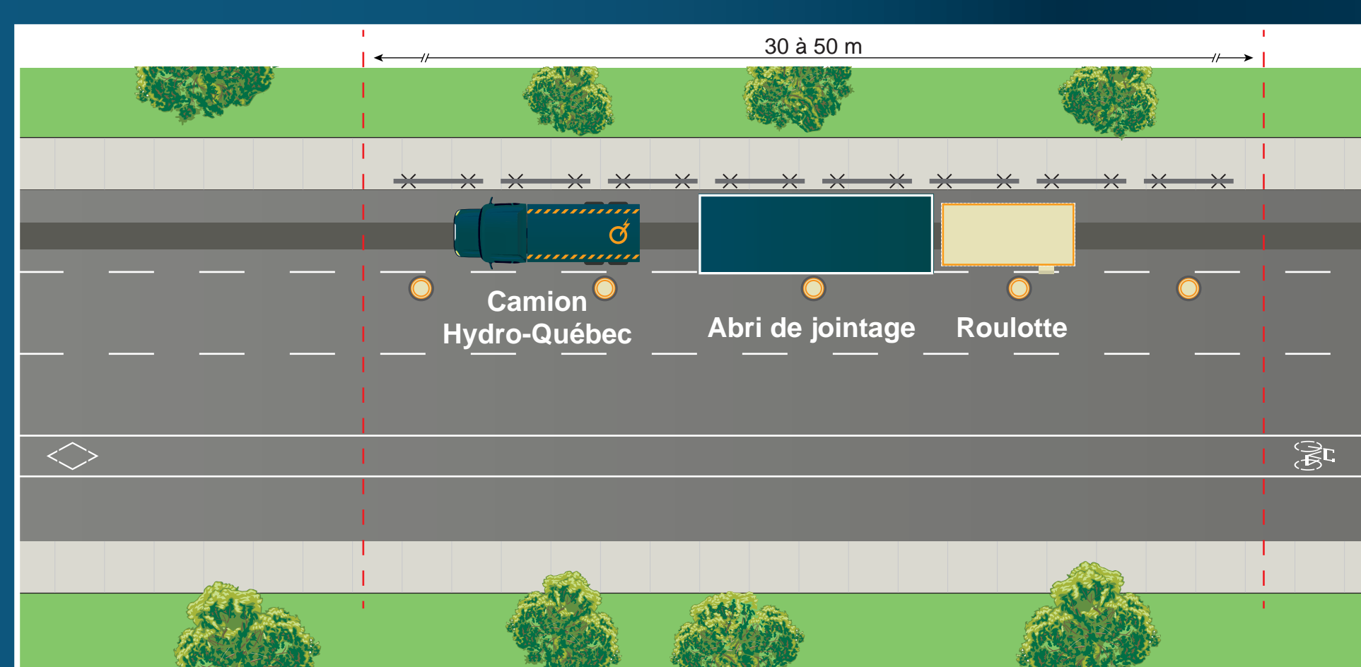
Étape 5 – Jointage des câbles, remblayage de la chambre et réfection des surfaces
