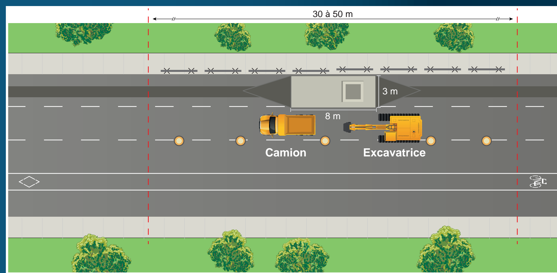
Étape 3 – Remblayage et installation du couvercle / réfection temporaire
