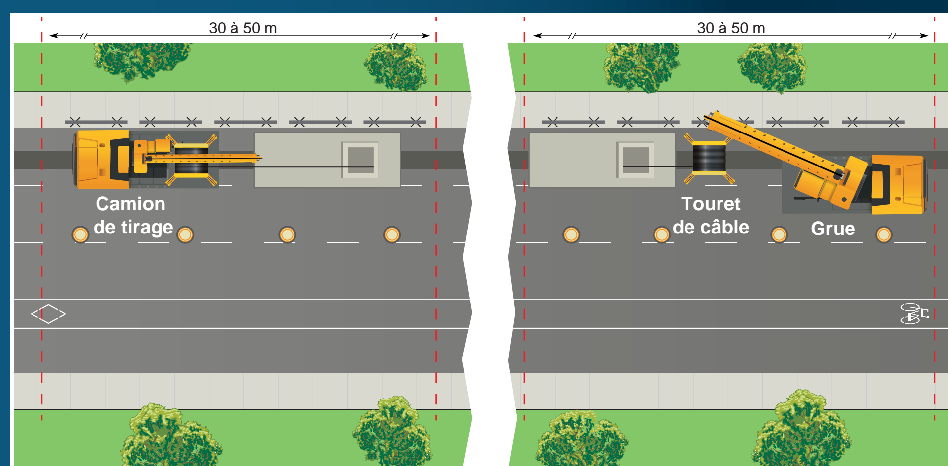
Étape 4 – Tirage des câbles
