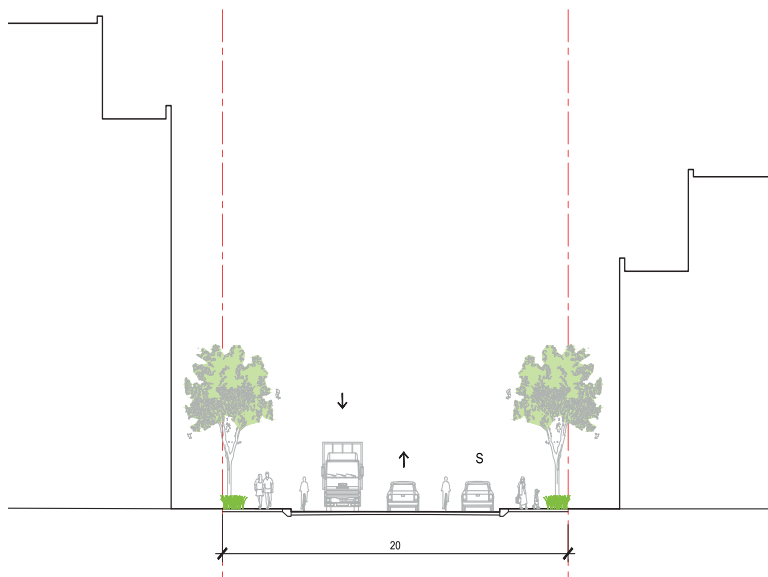
Coupe proposée de la rue de Marseille
