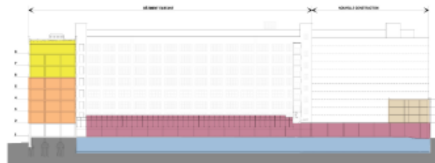
COUPE LONGITUDINALE, 2011
