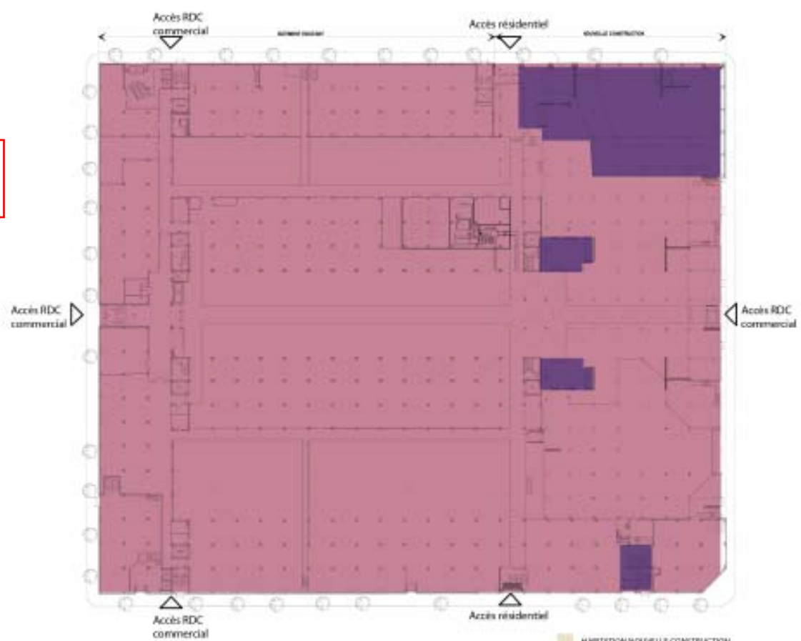
PLAN REZ-DE-CHAUSSÉE, 2011
