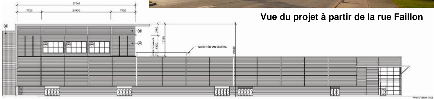
Élévation latérale est – rue Faillon
